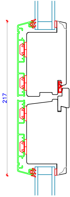
Samling, Halvdør
