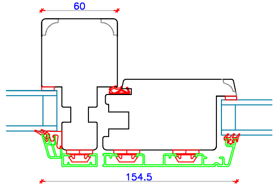
Lodpost/ ramme
