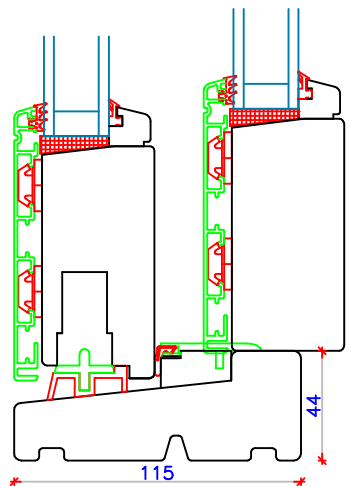
Trækarm/ enkelramme
