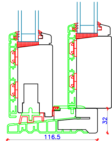
Træ-alukarm/ enkelramme
