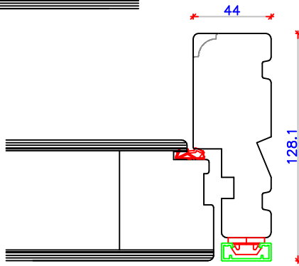
Sidekarm/ dørplade
