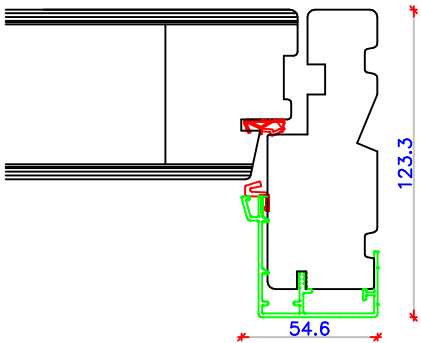
Sidekarm/ dørplade
