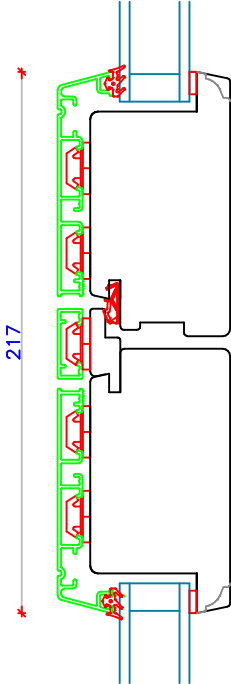
Samling, Halvdør
