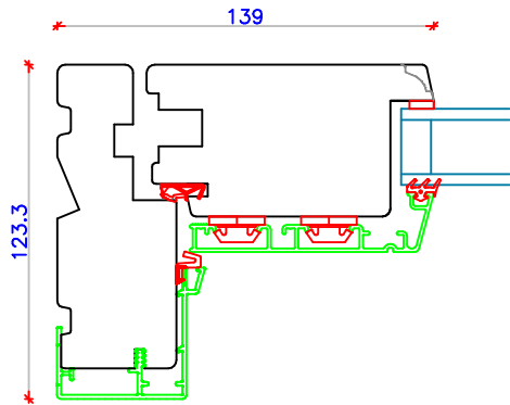
Sidekarm/ ramme
