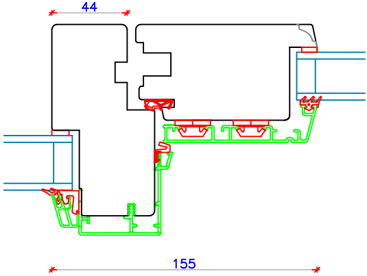
Lodpost/ ramme
