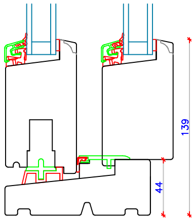
Trækarm/ enkeltramme
