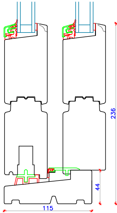
Trækarm/ dobbeltramme
