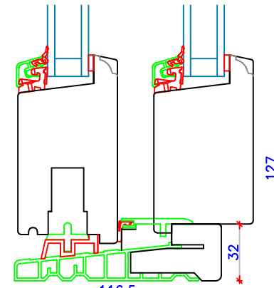
Træ-alukarm/ enkeltramme
