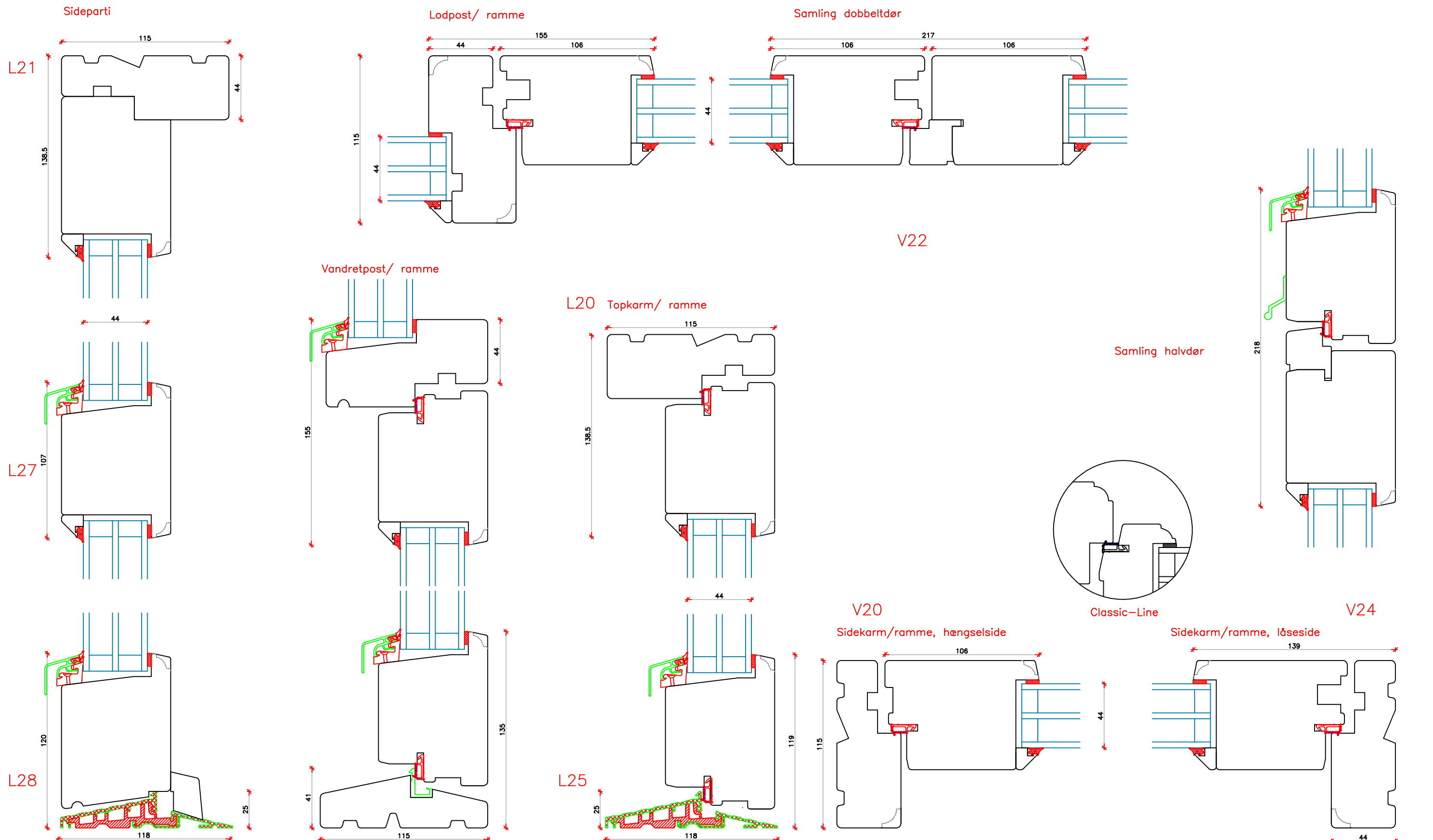
Hårdtræsbundstk.med aluskinne
