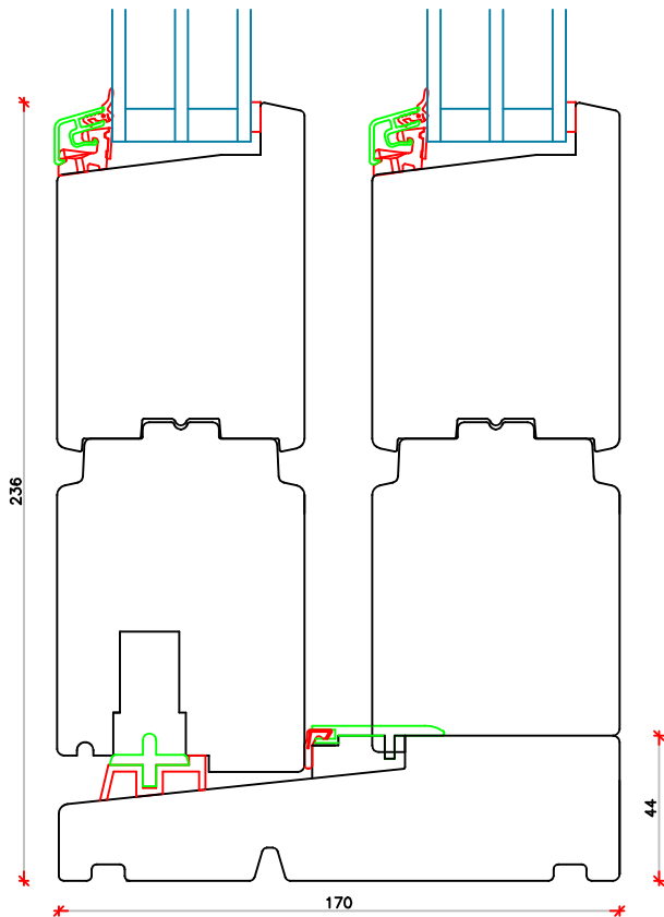
Hårdtræsbundtrin og dobbelt bundramme
